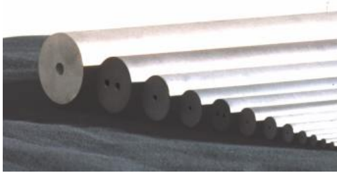
Rundstäbe Bohrungen gerade 1/2 Bohrungen, Länge bis 320 mm Durchmesser 1 mm – 40 mm
