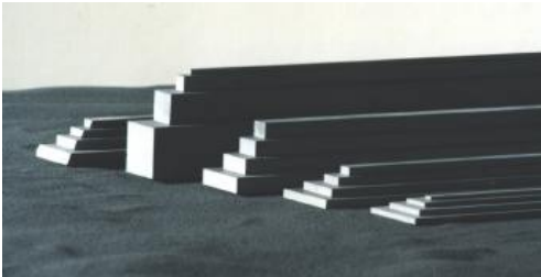
Rechteck-/Quadratstäbe Roh und geschliffen, Länge bis 320 mm Querschnitt 1x2 mm bis 8x40 mm
